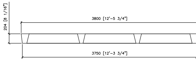
Elevation
